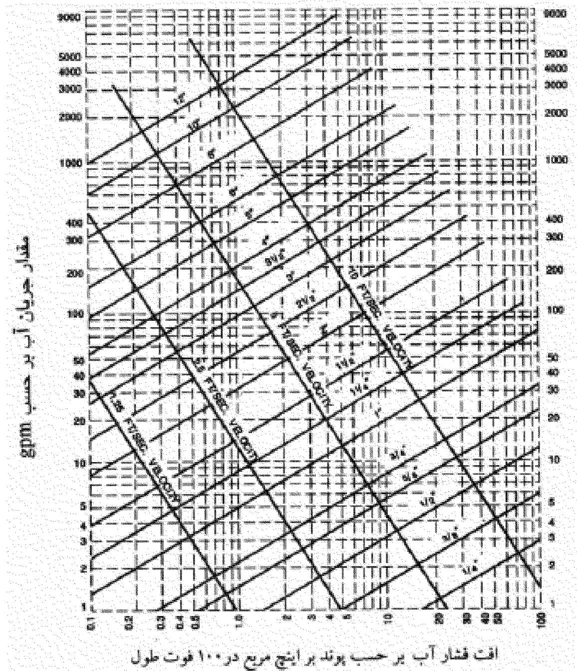
شکل پ ۱-۵-۵ (IP) منحنی اندازه گذاری لوله‌های مسی نوع K از استاندارد ANSI B 88
