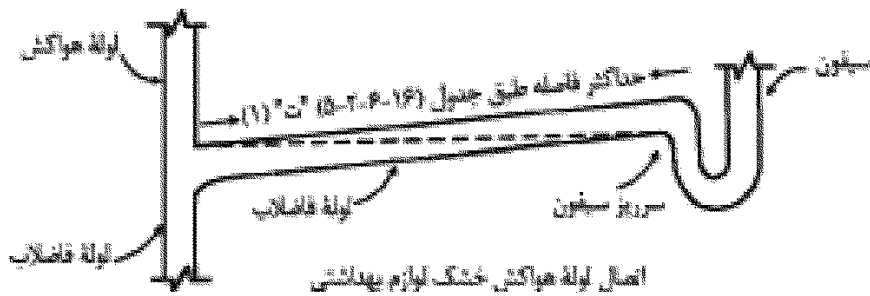
شکل شماره (۵-۲-۶-۱۶) "ت" (۱): اتصال لوله هواکش خشک لوازم بهداشتی
