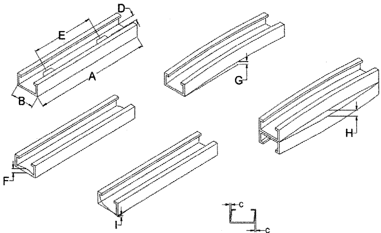
شکل ۱۱-۲-۱ رواداری ساخت اعضاء
