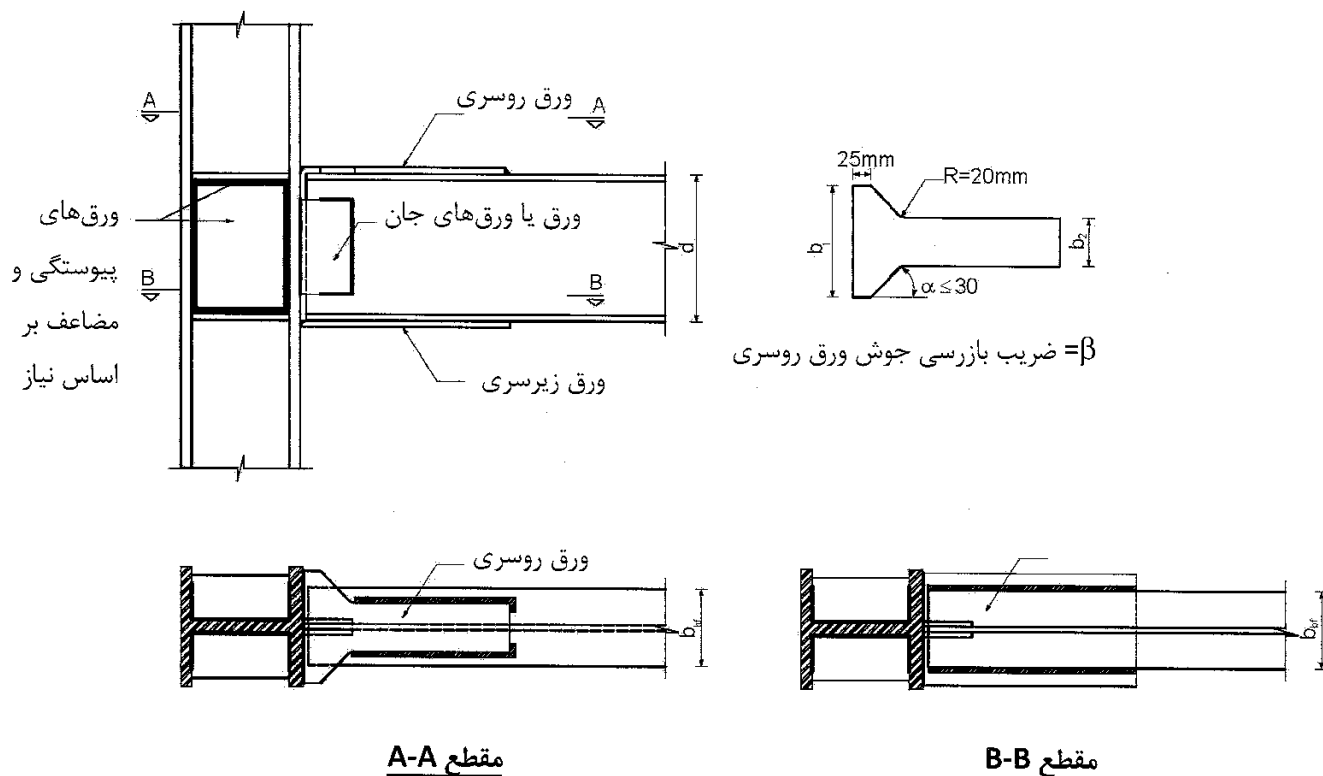
شکل ۱۰-۳-۱۰ اتصال گیردار جوشی به کمک ورق‌های روسری و زیرسری (WFP)
