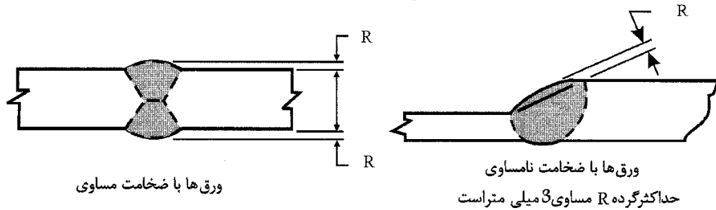
(ت) مقاطع قابل پذیرش جوش های شیاری
