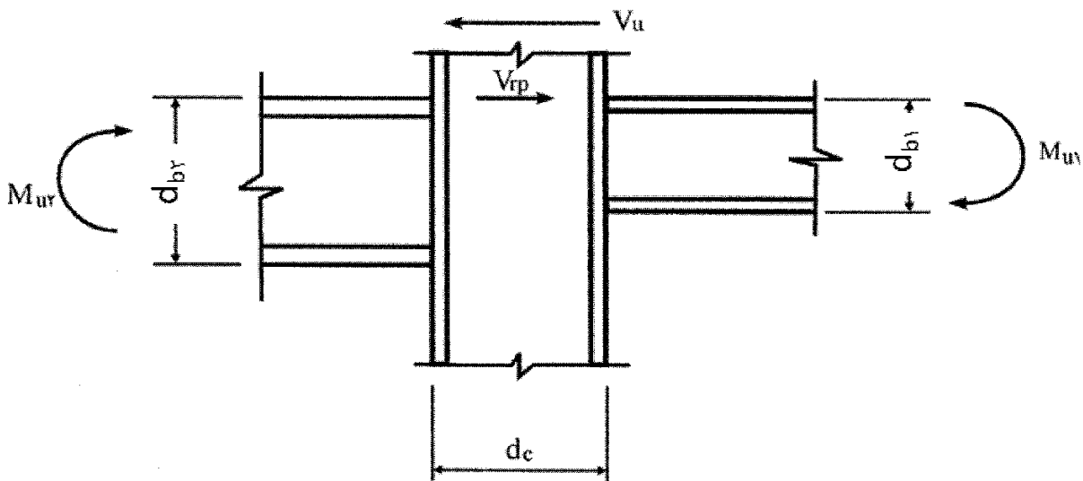
شکل ۲۱-۹-۲-۱۰ برش در چشمه اتصال
