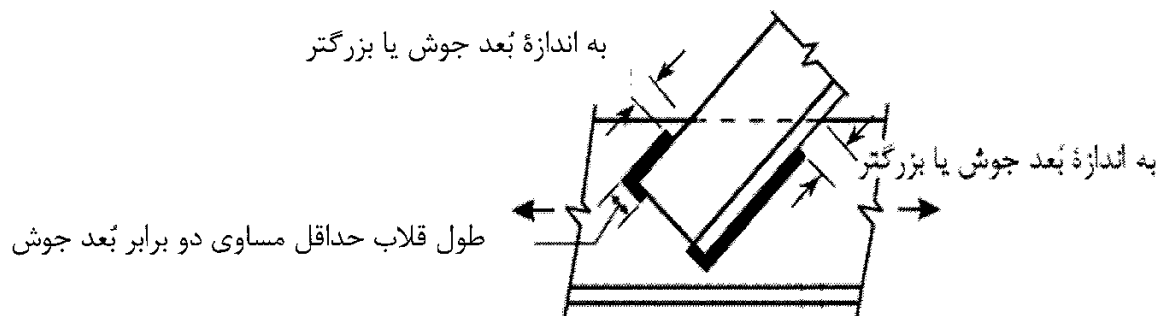
شکل ۱۰-۲-۹-۶ جوش گوشه در انتهای اعضای محوری
