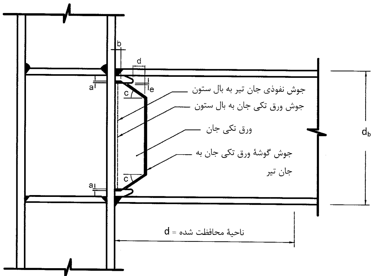
شکل ۱۰-۳-۱۳-۵ اتصال گیردار تقویت نشده جوشی (WUF-W)
