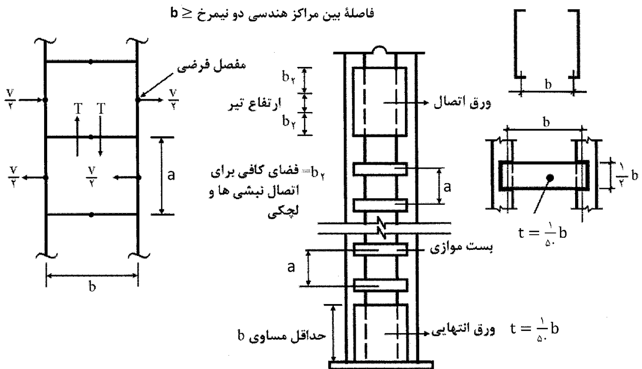
شکل ۱۰-۲-۴-۴ عضو فشاری ساخته شده با بست‌های موازی
