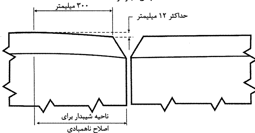
شکل ۲-۴-۱۰ اصلاح ناهمبادی و ناهم‌محوری
