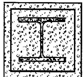
الف) عضو محوری مختلط محاط در بتن
