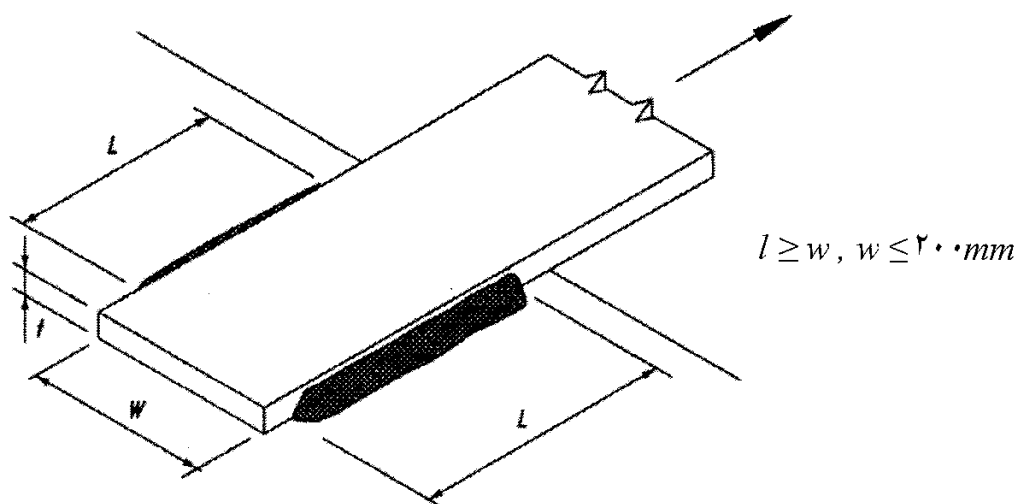
شکل ۱۰-۲-۹-۴ جوش گوشه در انتهای تسمه‌های کششی
