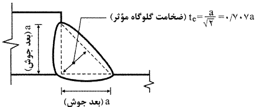
شکل ۱۰-۲-۹-۳ ضخامت گلوگاه موثر جوش‌های گوشه
