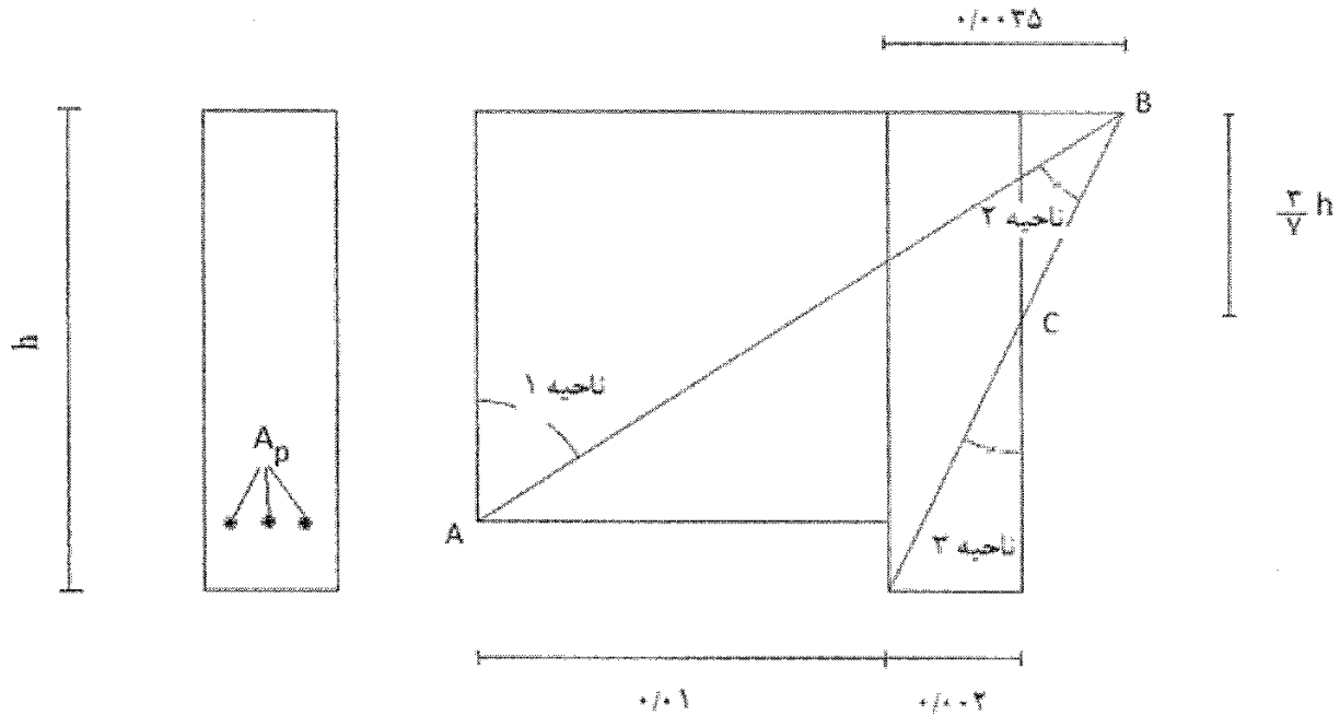
شکل ۹-۲۴-۱ نمودار تغییرشکل در حالت حدی نهایی
