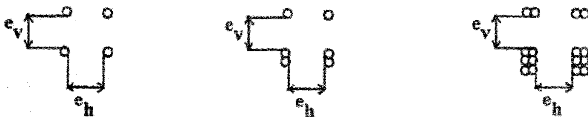
شکل ۲-۲۴-۹ دسته کردن کابل
